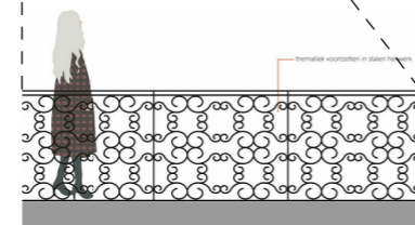
voorgevel
