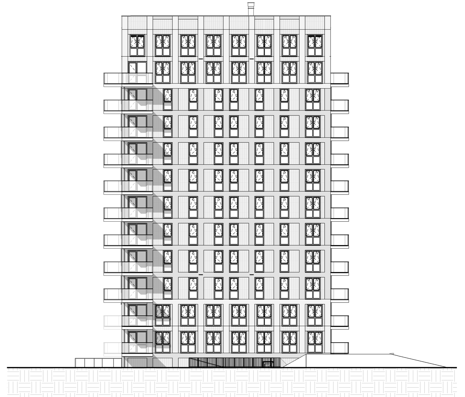
rechter zijgevel
